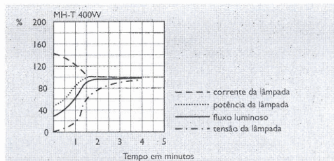
Performance da lâmpada na partida
